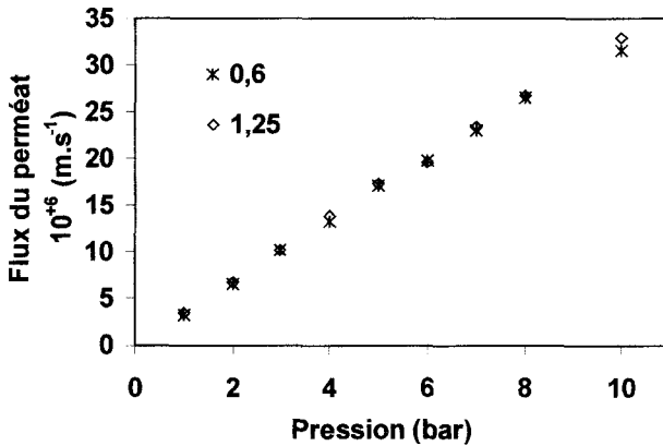
Figure 4 Effet de deux vitesses d'écoulement tangential (0,6 et 1,25 m·s -1 ) sur le flux du perméat d'une solution de NH 4 NO 3 (200 mg (NO 3 - )·L -1 ). Effect of two cross-flow velocities (0.6 and 1.25 m·s -1 ) on the permeate flux for a NH 4 NO 3 (200 mg (NO 3 - )·L -1 ) solution.
