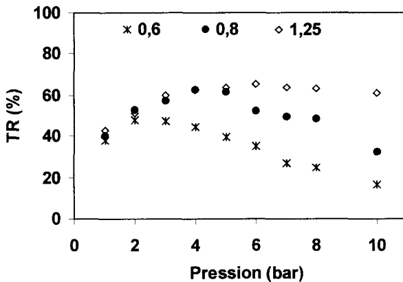
Figure 5 Effet de 3 vitesses d'écoulement tangential (0,6, 0,8 et 1,25 m·s -1 ) sur le taux de rétention d'une solution de NH 4 NO 3 (100 mg (NO 3 - )·L -1 ). Effect of three cross-flow velocities (0.6, 0.8 and 1.25 m·s -1 ) on the retention rate of a NH 4 NO 3 (100 mg (NO 3 - )·L -1 ) solution.
