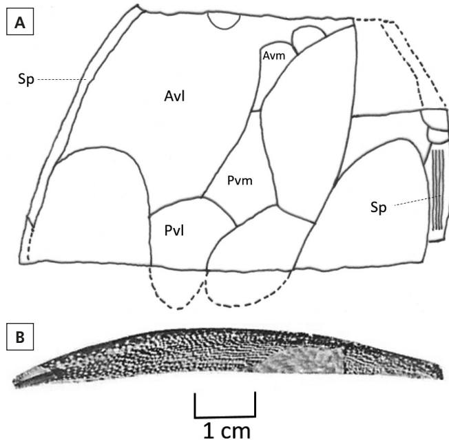
Figure 7. a) Schéma du bouclier thoracique du spécimen MHNM 02-11818a (Holotype Desbiensaspis yorki n. gen. n. sp.) de L'Anse-à-Brillant. Plaques : Avl (antéro-ventro-latérale), Avm (antéro-ventro-médiane), Pvl (postéro-ventro-latérale), Pvm (postéro-ventro-médiane), Sp (spinale). Dessin : Alexandra Pichet. b) Photo de la plaque spinale (Sp) d'un arthrodire ( Quebecaspis russelli n. gen. n. sp. Spécimen NMC-11143, Pageau, 1969b, p. 843, planche XXXII, fig. 4.) du gisement 6A de Cap-aux-Os montrant une ornementation tuberculée semblable à celle de la spinale de D. yorki .
