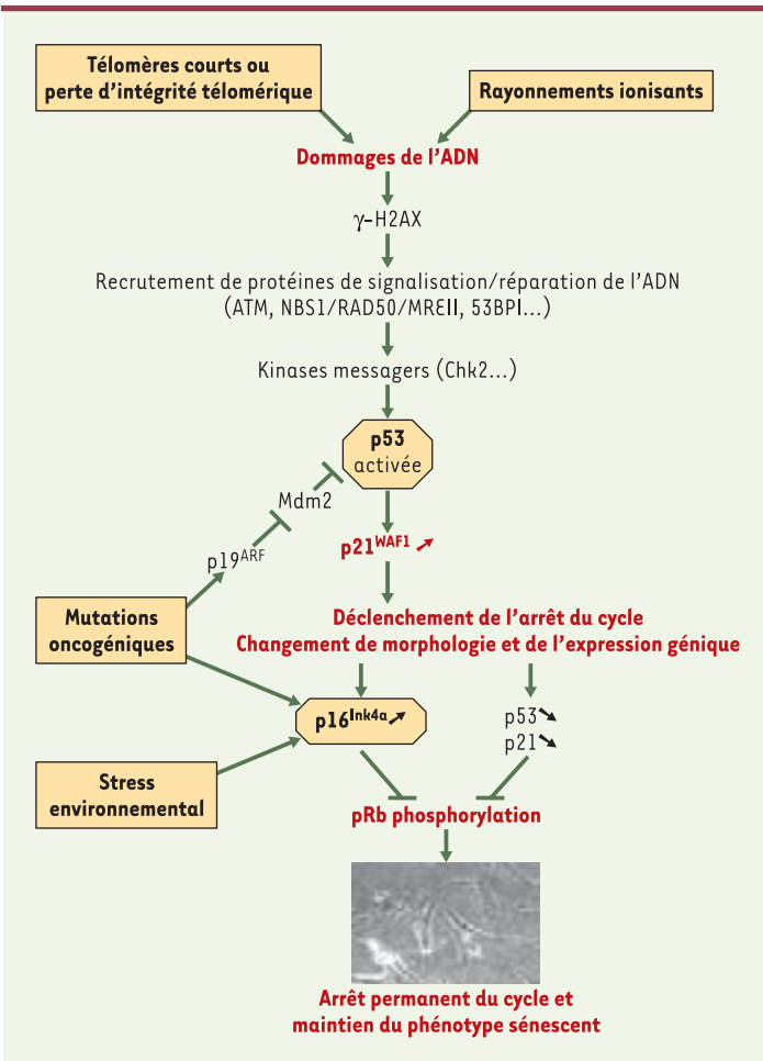
Figure 2. Mécanismes à la base de l'arrêt permanent du cycle cellulaire lors de la sénescence. Divers stimulus peuvent activer un programme commun de sénescence. Le raccourcissement des télomères est le stimulus physiologique le mieux décrit dans l'induction de la sénescence. L'expression d'oncogènes activés peut également déclencher la sénescence et représenterait une autre façon par laquelle la sénescence est un mécanisme suppresseur de tumeur. Le programme effecteur de la sénescence comprend les voies p53/p21 WAF1 et p16 INK4a /pRb. p53 serait activée par les kinases ATM/Chk2 (médiateurs des systèmes de réparation des dommages de l'ADN) ou par p19 ARF (médiateur de la voie signalétique activée par ras oncogénique chez la souris). Le facteur p16 INK4a serait activé par le stress imposé par des conditions inadéquates de culture et par une stimulation oncogénique dérégulée. Les mécanismes responsables de l'accumulation de p16 INK4a sont encore méconnus.
