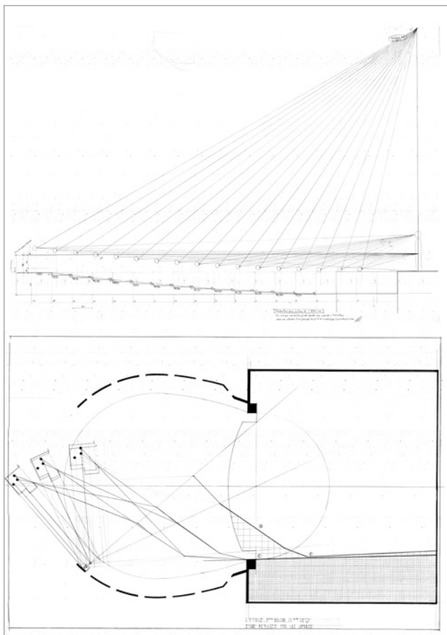
FIG. 19. STUDIES OF VIEWS DATED FROM SEPTEMBER 1989. SECTION OF LAYOUT FOR PARTERRE, WHICH READS: "CECI N'EST PAS UNE SOLUTION FINALE LAQUELLE SERA RAFFINÉE À L'ORDINATEUR, MAIS UNE INTENTION ET UN PRINCIPE TRÈS PROCHE DE LA RÉALITÉ QUE L'ON VOUDRAIT VOIR" (TOP). SKETCH PLAN OF THE 21 ST SEAT ON BALCONY 3 LEVEL (BOTTOM). | ARCHIVES LUC LAPORTE.
