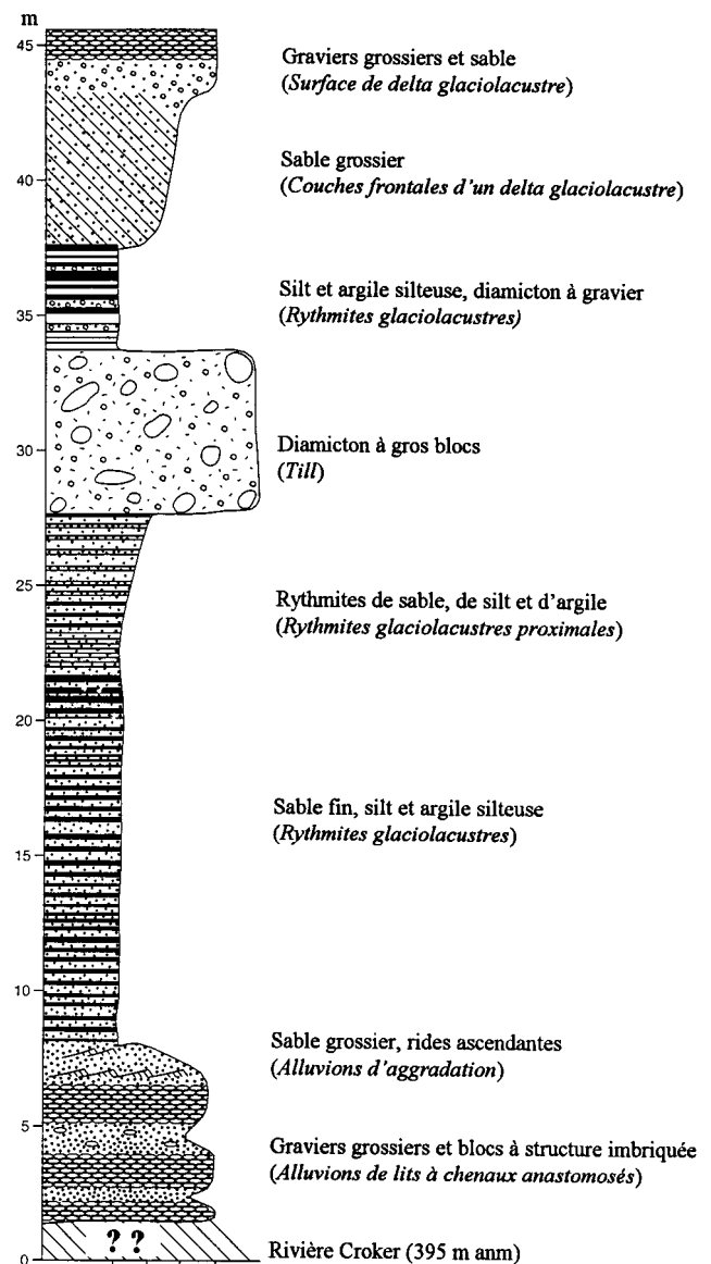
FIGURE 2. Coupe composite de la séquence de sédiments exposés sur le versant est de la rivière Croker (voir 1, fig. 1). Interprétation génétique en italique.
