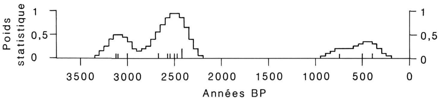
FIGURE 4. Histogramme des poids statistiques des dates 14 C des sols enfouis (traitement statistique selon la méthode proposée par OCCHIETTI et HILLAIRES-MARCEL, 1977).
