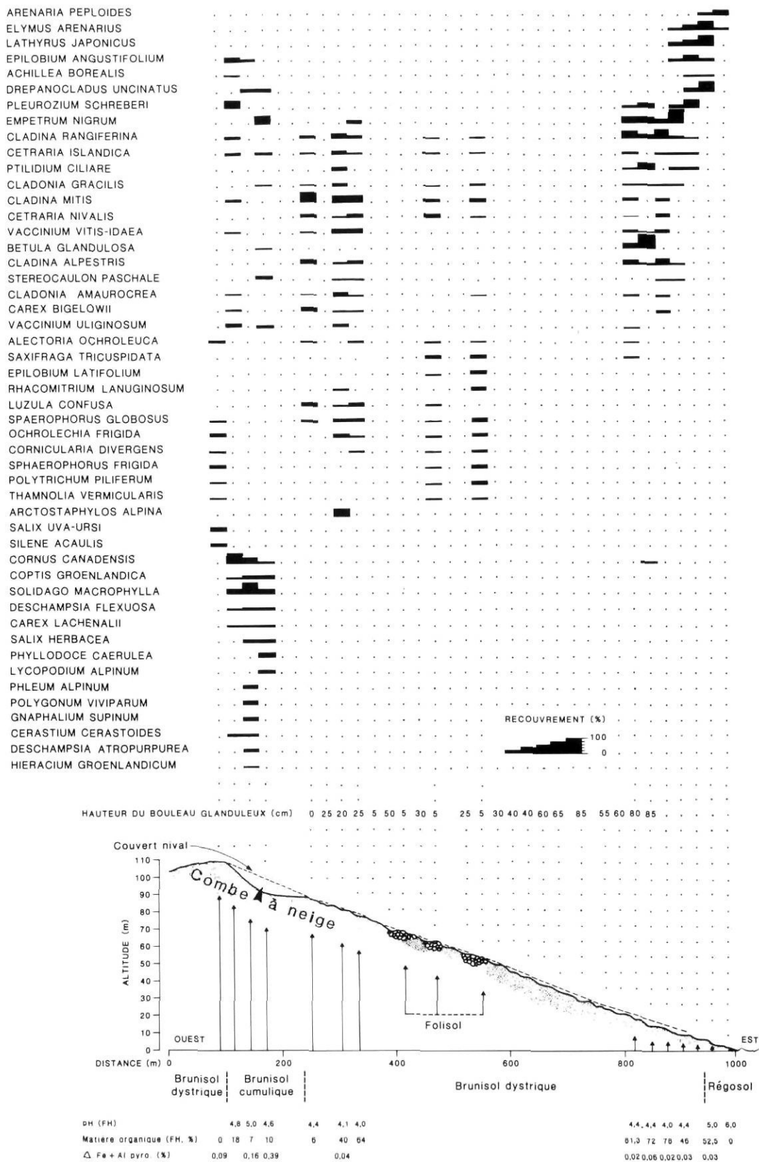
FIGURE 2. Toposéquence de la végétation et des sols de la vallée étudiée et conditions d'enneigement.
