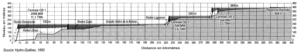
Figure 2 Le projet Grande-Baleine. Localisation des barrages et centrales
