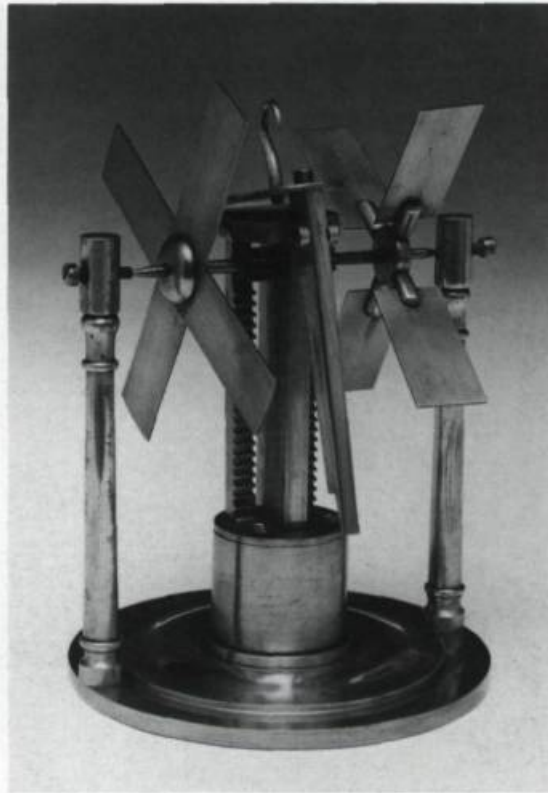
Moulinet servant à montrer la résistance de l'air en usage au cabinet de physique créé en 1806 par Jérôme Demers et Félix Gatien. Photo: Kedl. (Musée du Séminaire de Québec).
