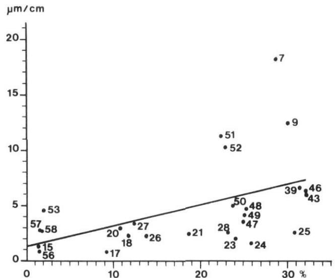
FIGURE 11. Corrélation entre la porosité (%) et l'augmentation de longueur (micromètres/cm) de tous les échantillons étudiés. Coefficient de corrélation : 0,49, significatif au seuil de 5 %.
