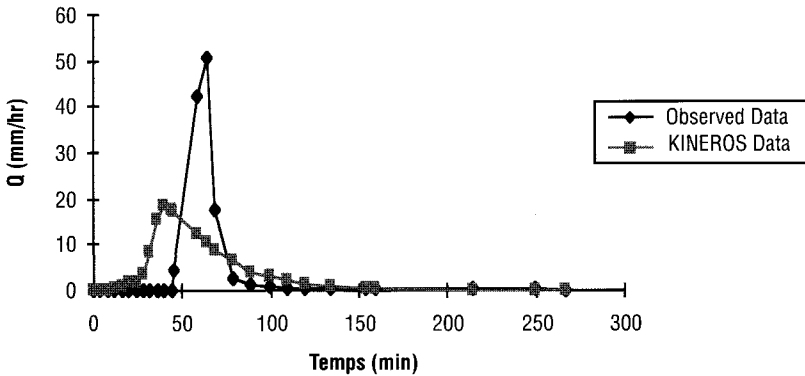
Figure 3 Hydrogrammes Mesuré et Simulé par le Modèle KINEROS (averse du 24/09/95). Measured and KINEROS simulated hydrographs (rainstorm of the 24/09/95).
