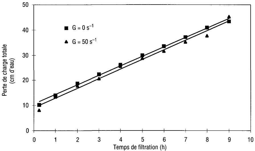
Figure 8 Variation de la perte de charge en fonction du temps de filtration pour G = 0 et G = 50 \text{ s}^{-1} ( V_f = 5 \text{ m/h} ; A/P = 2 ; T_f = 10 \text{ mn} ; \text{pH} = 6,5 ; C_p = 2 \text{ mg/l} ).
