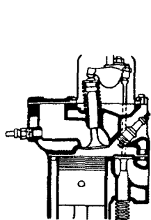
Moteur à soupapes en tête et arbre à cames dans le carter
