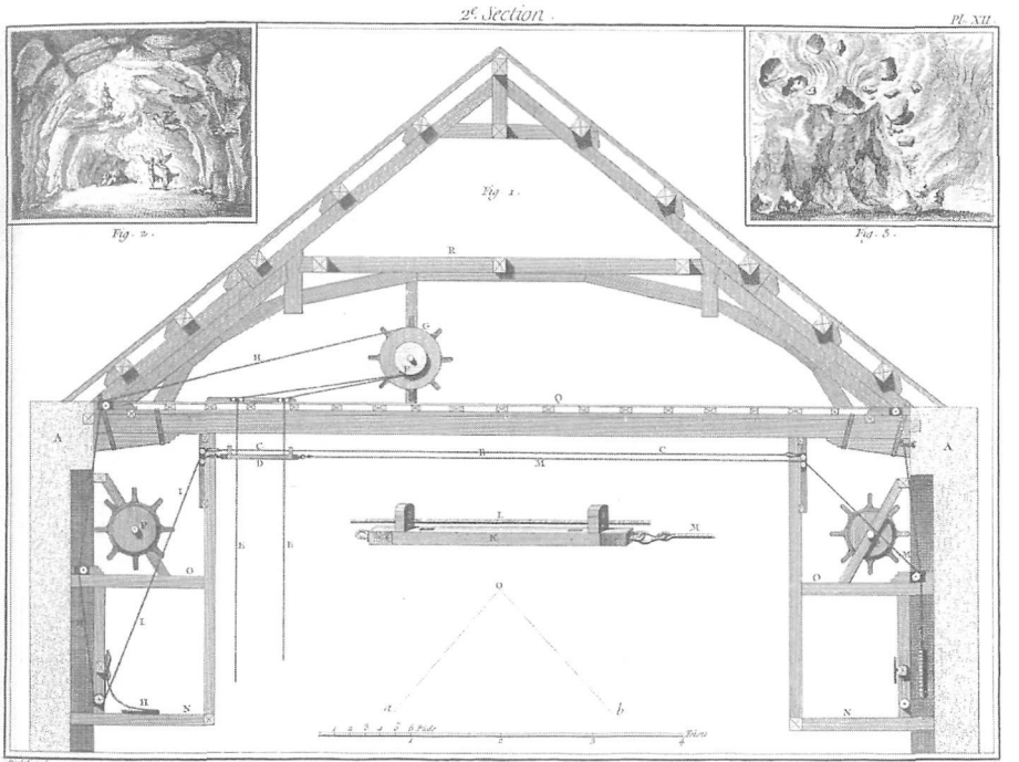
Machines de Théâtres. Élévation en Coupe de la charpente du Comble et des corridors avec le Développement d'une Machine de Travers, et abstraction en esquisse de Descriptions d'un autre système et d'un bâton réglant.
