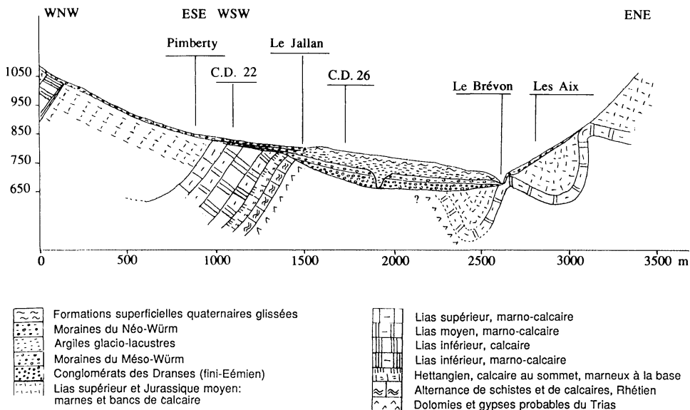
COUPE INTERPRÉTATIVE DU VERSANT DE VAILLY (Secteur de Pimberty-Le Lavouet)
