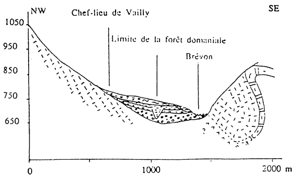
COUPE INTERPRÉTATIVE DU VERSANT DE VAILLY (500 mètres à l'aval du précédent)
