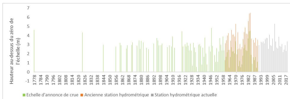
Figure 4 : Hauteurs de crue aux différentes échelles de Malzéville
