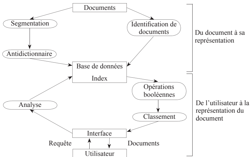
Fig. 1 : Schéma général d'un moteur de recherche
