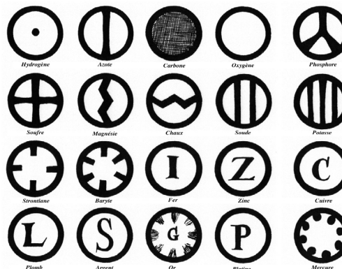
Figure 14. Symboles chimiques selon Dalton (1806).
