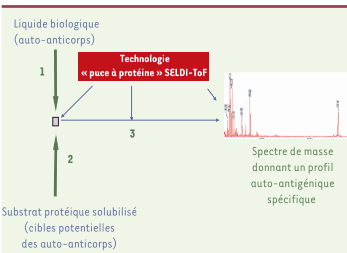
Figure 3. Technologie SELDI ( surface-enhanced laser desorption/ionisation ). La solution d'auto-anticorps à analyser est incubée avec une puce à protéine A, fournie par Ciphergen, qui a la propriété de fixer spécifiquement les immunoglobulines de classe G. Cette puce à anticorps est ensuite incubée avec une solution contenant les protéines susceptibles d'être les cibles des auto-anticorps (étape 2). Les auto-antigènes, fixés sur la puce de manière non ordonnée, peuvent cependant être rangés dans l'ordre de leur masse moléculaire en appliquant directement sur la puce la technologie de spectrométrie de masse SELDI-ToF ( time of flight ) (étape 3).
