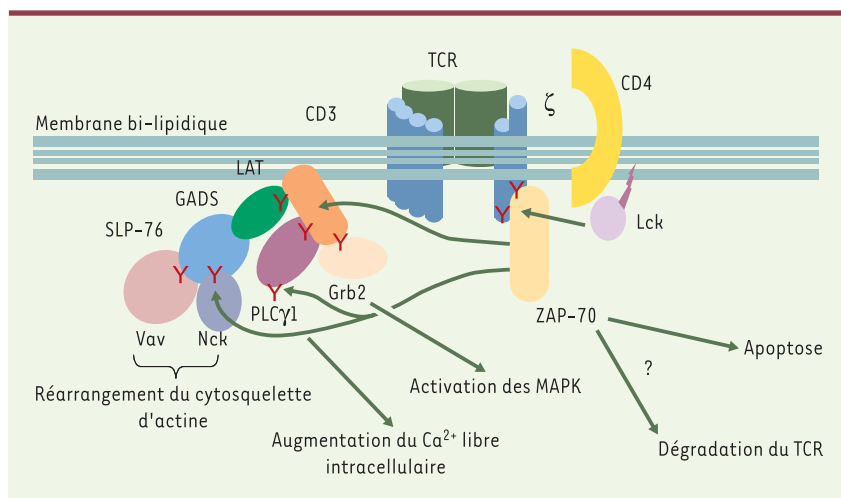
Figure 3. Voies de signalisation contrôlées par ZAP-70. Après stimulation du TCR, la tyrosine kinase p56 Lck ( lymphoid cell kinase ), associée à la face interne de la membrane, phosphoryle des résidus tyrosine (Y) présents dans les molécules CD3 et ζ. Cette phosphorylation permet le recrutement de ZAP-70, qui est alors phosphorylée par p56 Lck et activée. ZAP-70 phosphoryle à son tour LAT sur plusieurs tyrosines. Une fois phosphorylées, ces tyrosines servent d'ancrage à d'autres protéines de signalisation qui sont elles-mêmes phosphorylées et activées, permettant le remaniement du cytosquelette d'actine, un signal calcique et l'activation des MAPK. La fin de la réponse T est également contrôlée par ZAP-70, qui est nécessaire à l'apoptose et à la dégradation du TCR induites par stimulation de ce récepteur. LAT: linker for activation of T cells ; SLP76: SH2-containing leukocyte protein of 76 kDa ; GADS: Grb2-related adapter downstream of Shc ; Grb2: growth factor receptor bound protein 2 ; PLCγ1: phospholipase C; MAPK: mitogen-activated protein kinase .
