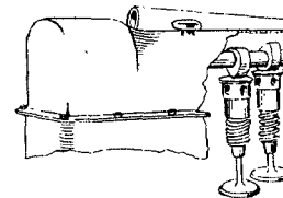
Moteur à soupapes bilatérales
