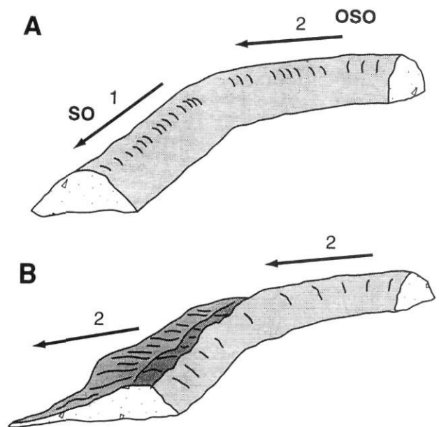
FIGURE 6. A) Forme fuselée hypothétique, dont la crête de la moitié aval (1) est tournée vers le SO et celle de la moitié amont (2) vers l'OSO, en raison d'un changement dans le sens d'écoulement des glaces à l'est de la baie James selon Hardy (1976). B) Morphologie probable de la partie aval de la forme fuselée par suite du changement dans le sens de l'écoulement régional passant du SO à l'OSO.
