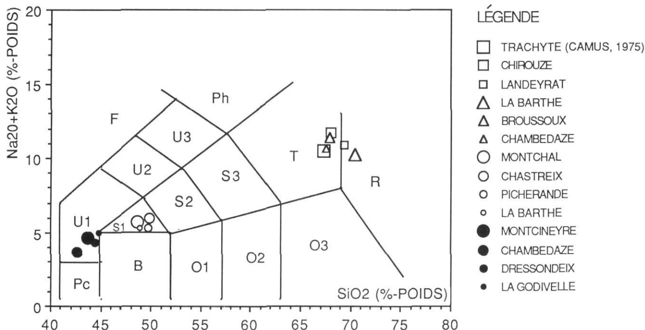
FIGURE 2. Détermination des magmas selon la classification de Le Bas et al. (1985) de trois téphras présentes dans des tourbières de l'Artense, du Cézalier et du NE du Cantal. Explication : F, foïdite ; Pc, picrobasalte ; U1, basanite, si Ol_{nr} > 10\% ou téphrite, si Ol_{nr} \leq 10\% ; U2, phonotéphrite ; U3, téphriphonolite ; Ph, phonolite ; B, basalte alcalin ; O1, andésite basaltique ; O2, andésite ; O3, dacite ; R, rhyolite ; S1, trachybasalte : hawaïte si (Na_2O-2) \geq K_2O (%-p) ou trachybasalte potassique si (Na_2O-2) < K_2O ; S2, trachyandésite basaltique ; S3, trachyandésite ; T, trachyte, si Q_{nr} \geq 20\% , ou trachydacite, si Q_{nr} \leq 20\% . Les parts de silice et d'alcalins sont celles du tableau I.
