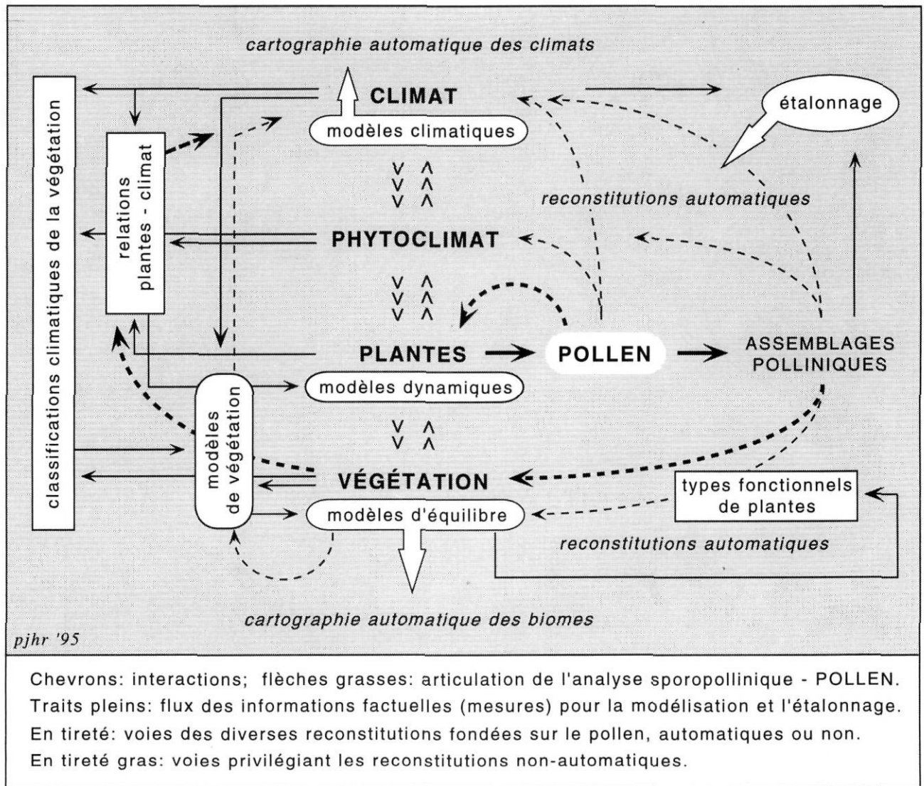
FIGURE 2. Articulation de l'analyse pollinique dans l'étude du système climatique. Les assemblages polliniques actuels ou anciens sont dérivés du pollen produit par des plantes qui subissent un phytoclimat local à chaque stade de leur cycle vital. Climat, phytoclimat, plantes et végétation agissent les uns sur les autres à des échelles variées. Les rectangles matérialisent les typologies et les classifications; les parallélogrammes à bouts arrondis et l'ellipse correspondent aux modèles et à l'étalonnage par des fonctions mathématiques.
