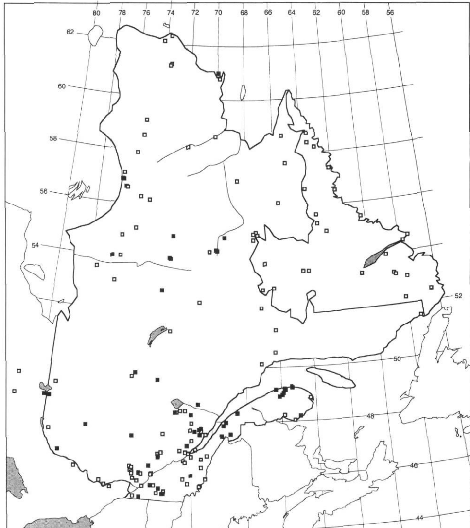
FIGURE 5. Localisation des données polliniques disponibles pour la période des 6000 ans BP (carrés blancs). Carrés noirs : données disponibles aussi pour les charbons de bois microscopiques.
