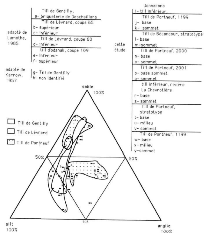
FIGURE 5. Analyses granulométriques de la matrice de différents tills pré-Saint-Pierre de la vallée du Saint-Laurent.
