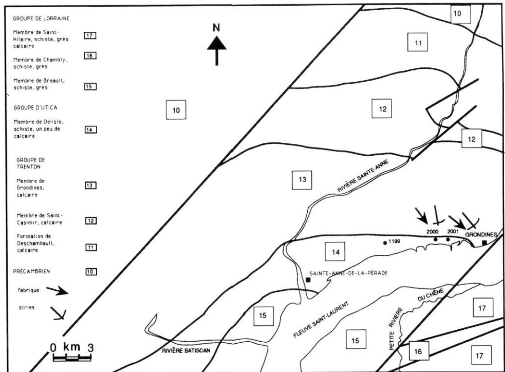
FIGURE 2. Carte géologique simplifiée de la région de Sainte-Anne-de-la-Pérade.
