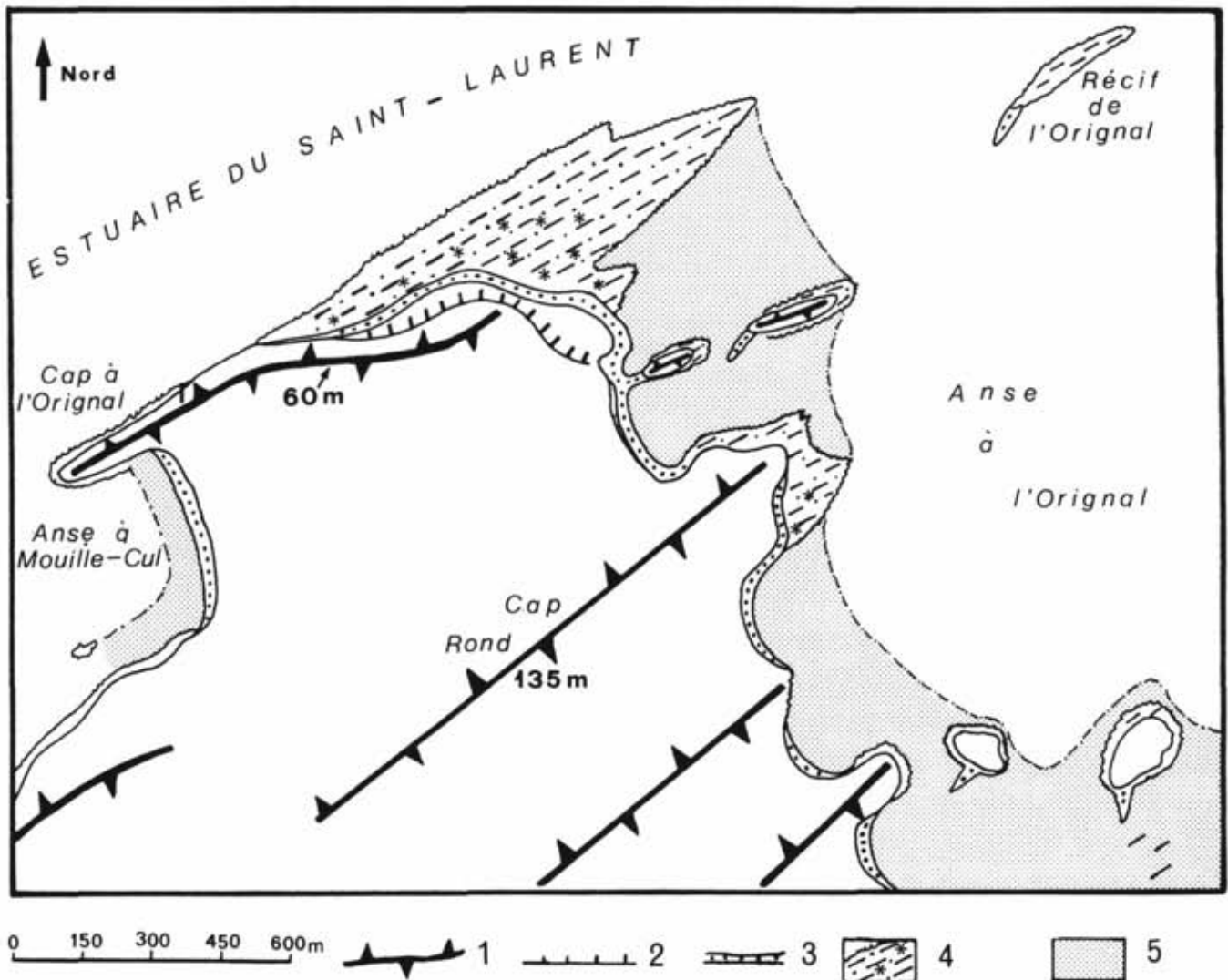
FIGURE 7. Promontoire de l'Original. Légende des signes: 1) crête appalachienne; 2) falaise Mitis (Mic Mac); 3) cordon littoral; 4) estran rocheux (étoiles: cryoplanation; points: éléments détritiques); 5) estran sablo-vaseux.
