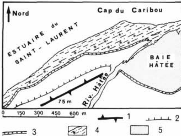
FIGURE 8. Cap du Caribou. Légende des signes: 1) crête appalachienne; 2) falaise Mitis (Mic Mac); 3) cordon littoral; 4) estran rocheux (étoiles: cryoplanation; points: éléments détritiques); 5) estran sablo-vaseux. Cap du Caribou. Captions: 1) Appalachian ridge; 2) Mitis (Mic Mac) cliff; 3) high water ridge; 4) rocky platform (stars: cryoplanation; dots: loose particles); 5) sand and silt.
