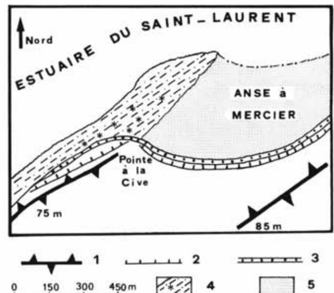
FIGURE 5. Pointe à la Cive. Légende des signes ; 1) crête appalachienne ; 2) falaise Mitis (Mic Mac) ; 3) cordon littoral ; 4) estran rocheux (étoiles : cryoplanation ; points : éléments détritiques) ; 5) estran vaseux.
