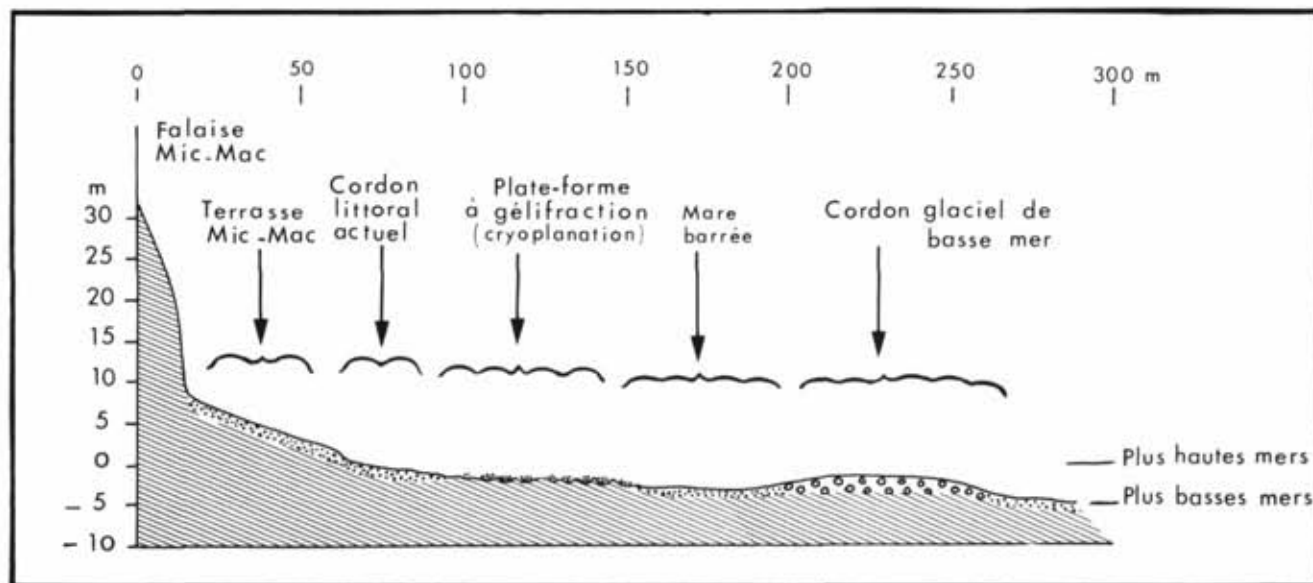
FIGURE 13. Sacré-Cœur de Rimouski. Profil de l'étagement.
