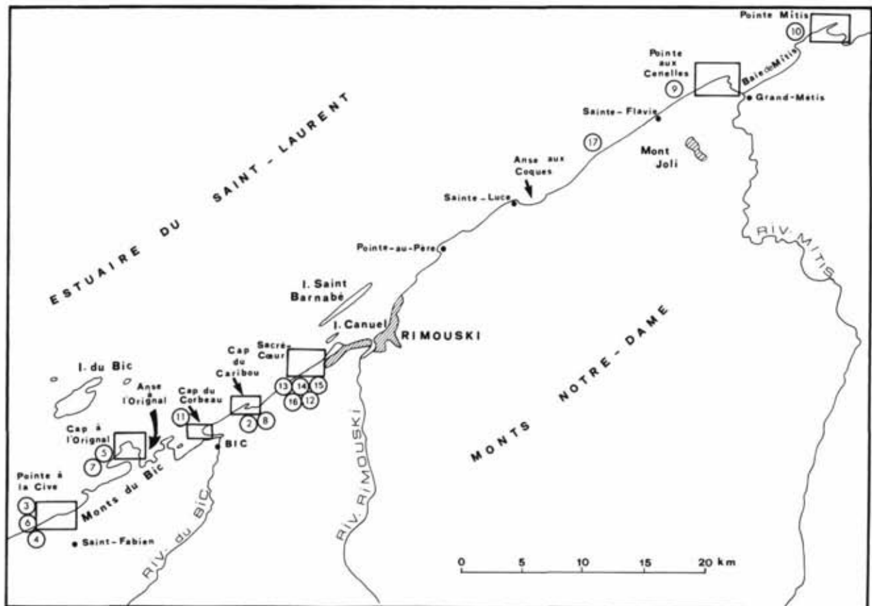
FIGURE 1. Localisation générale des lieux d'étude dans la région de Rimouski. Encadrements: emplacements des figures au trait et des photos, avec leurs numéros.
