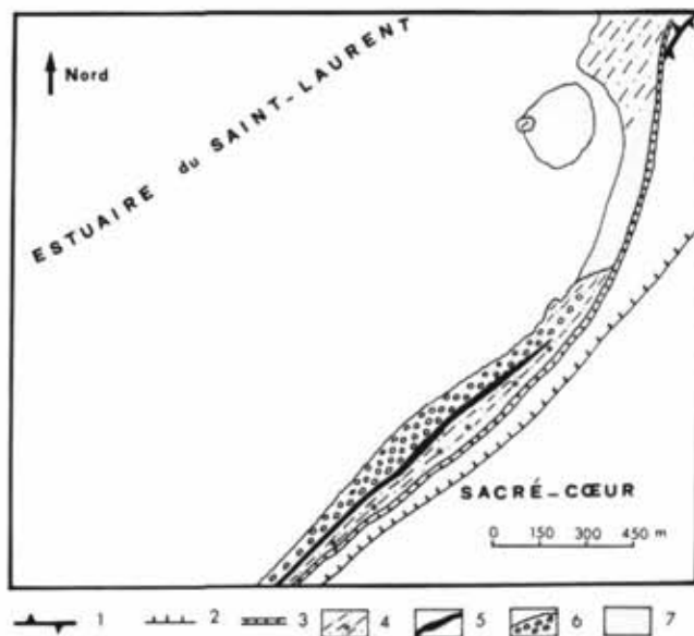
FIGURE 12. Sacré-Cœur de Rimouski. Carte de l'étagement. Légende des signes: 1) crête appalachienne; 2) falaise Mitis (Mic Mac) et terrasse à son pied; 3) cordon littoral de haute mer; 4) estran rocheux de cryoplanation (étoiles: cryoplanation; points: éléments détritiques); 5) mare longitudinale barrée; 6) cordon glaciaire de basse mer; 7) estran sablo-vaseux.
