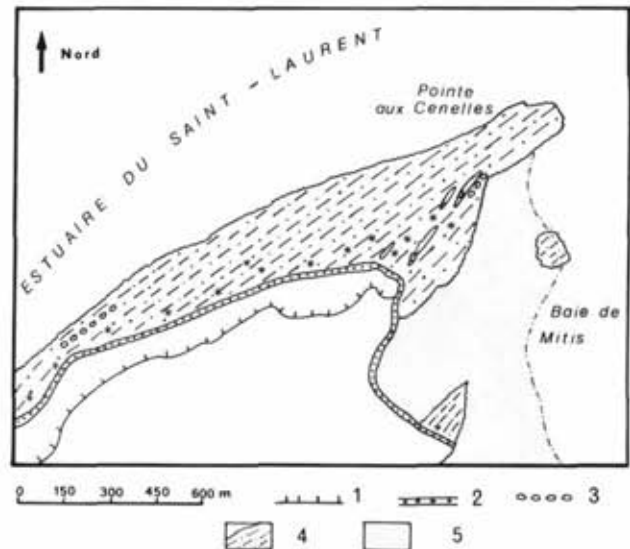
FIGURE 9. Pointe aux Cenelles. Légende des signes: 1) Falaise Mitis (Mic Mac); 2) cordon littoral; 3) cordon glacial de basse mer; 4) estran rocheux (étoiles: cryoplanation; points: éléments détritiques); 5) estran sablo-vaseux. Pointe aux Cenelles. Captions: 1) Mitis (Mic Mac) cliff; 2) high water ridge; 3) boulder barricade; 4) rocky platform (stars: cryoplanation; dots: loose particles); 5) sand and silt.
