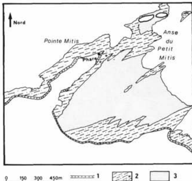
FIGURE 10. Pointe Mitis. Légende des signes: 1) cordon littoral; 2) estran rocheux (étoiles: gélifraction; points: éléments détritiques); 3) estran sablo-vaseux.
