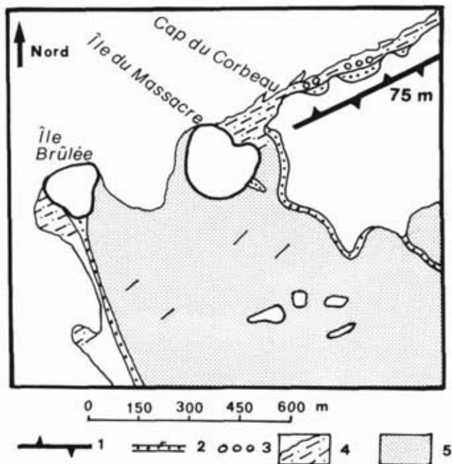
FIGURE 11. Cap du Corbeau. Légendes signes: 1) crête appalachienne; 2) cordon littoral et queue en position d'abri; 3) cordon glaciaire de basse mer; 4) estran rocheux; 5) estran sablo-vaseux.
