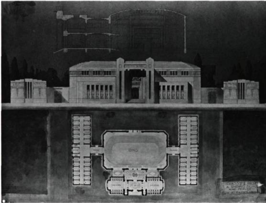
«A Riding School, class «B» II project.» Plan, élévation, coupe. Mine, encre et lavis sur canevas, 79 cm x 102 cm.
