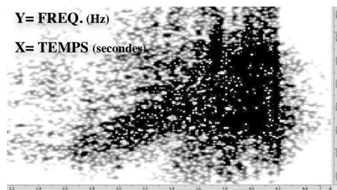
FIGURE 3 Analyse d'un cri de chouette effraie en vol.
