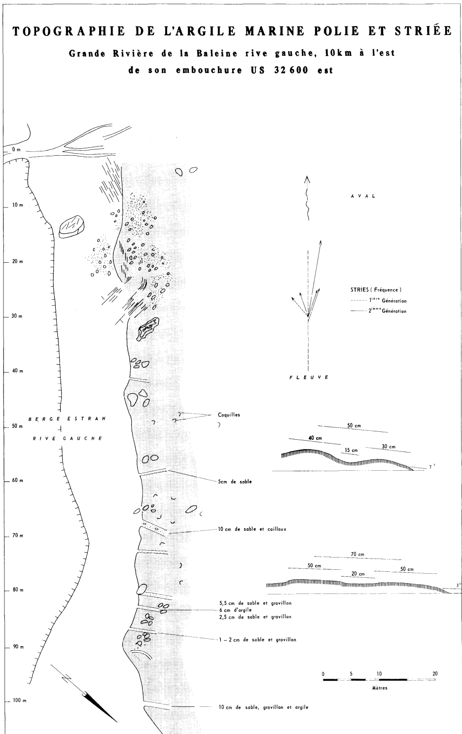
Figure 5 Topographie de l'argile marine polie et striée.
