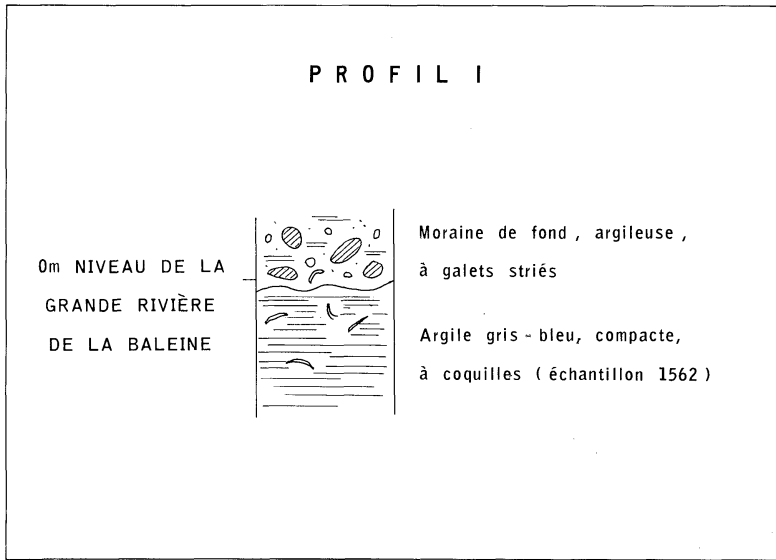
Figure 2 Profil I (P1). Contact de moraine de fond sur argile marine près de l'embouchure de l'affluent A, au niveau du fleuve (figure 1, p1). Les profils P2 et P3 ont été relevés plus haut sur la berge et plus en aval. 15 juillet 1969.
