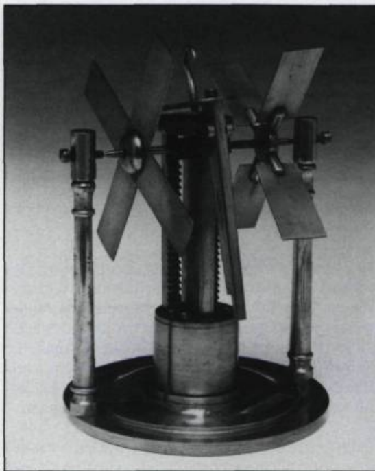
Moulinet servant à montrer la résistance de l'air en usage au cabinet de physique créé en 1806 par Jérôme Demers et Félix Gatién. (Photo: Kedl, Musée du Séminaire de Québec).
