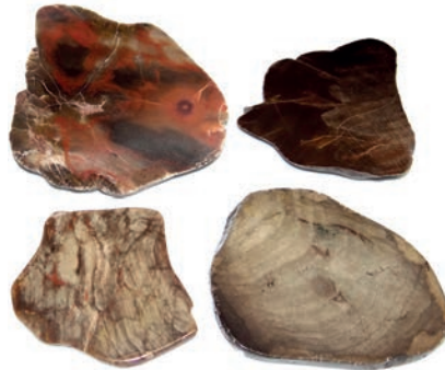
Trancher les pierres permet de voir leur composition intérieure. Collection Jocelle Cauvier
